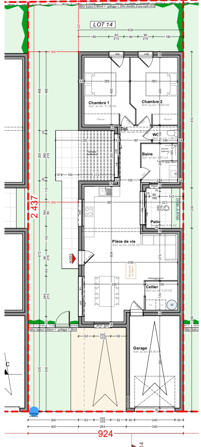
Plan de niveau - Rez de Chaussée - 1/100e
