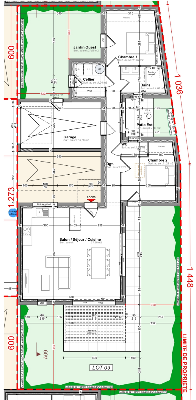
Plan de niveau - Rez de Chaussée - 1/100e
